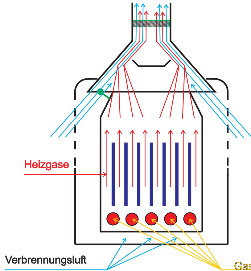
Aufstrom im Abgasstutzen
